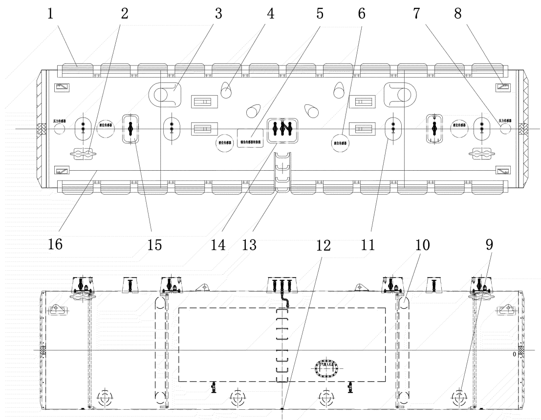
图 2 浮筒组成示意
