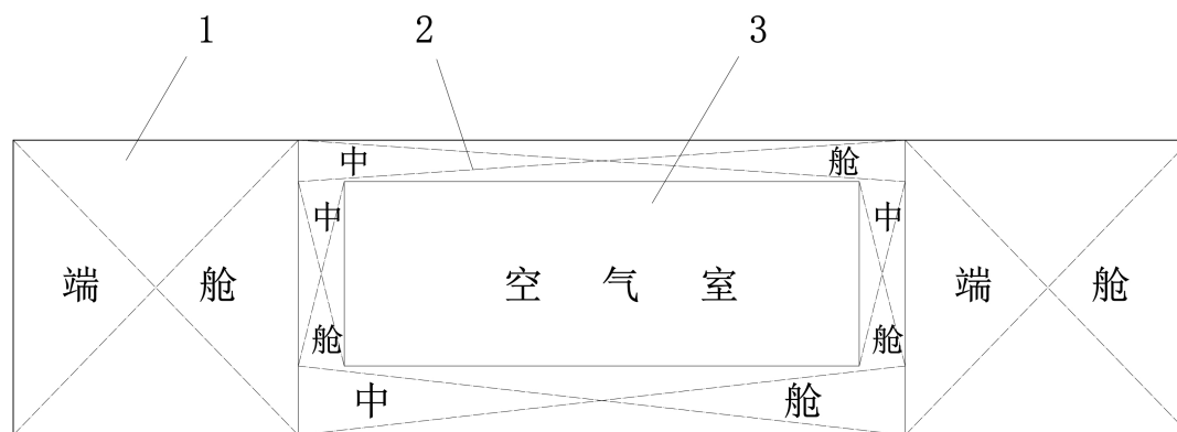
图1 浮筒结构示意图
