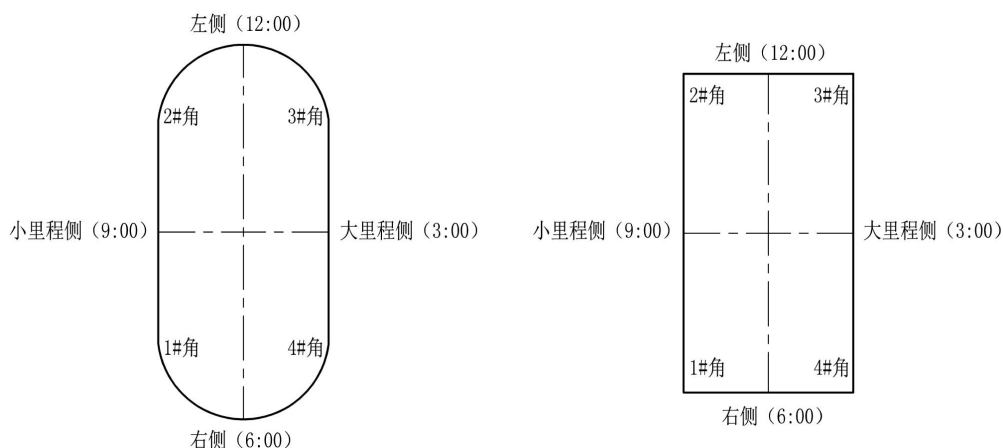
图 1.1 圆端形、矩形桥墩方位图
