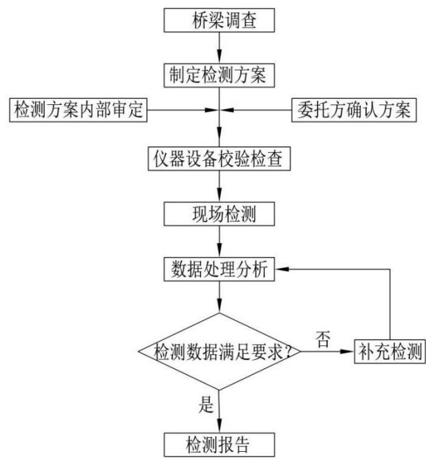
图 1 检测工作流程图
